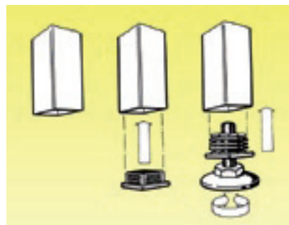
Standardfuß. Mitte. Nivellierfuß. Rechts. Optional zum Ausgleich kleiner Unebenheiten.
