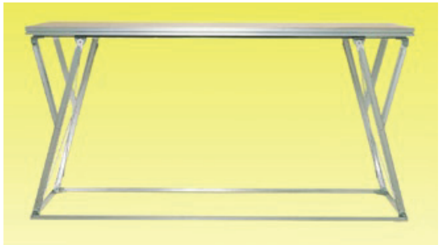
Version NIVOflex®-Gigant. Abmessungen 3 x 1 m für Höhen bis 150 cm.
