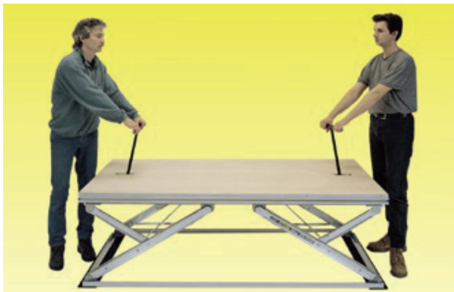
Die Versionen NIVOflex®-Comfort und NIVOflex®-AirStage für den Festeinbau werden von oben betätigt. Siehe Prospekt „Saalbodenverstellungen, manuell“.
